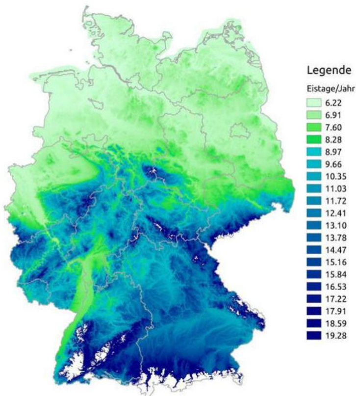
Abbildung 2.4.1: Eistage pro Jahr basierend auf /1.8/ für Höhen bis 700m üNN.
